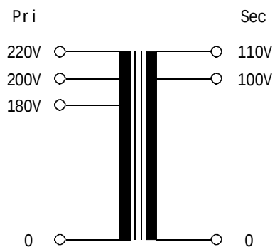
結線図
